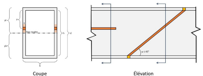
Situation #8 : Tubes rectangulaires assemblés avec soudures obliques considérées comme longitudinales ; Extrusions en « C » assemblées avec des soudures longitudinales
