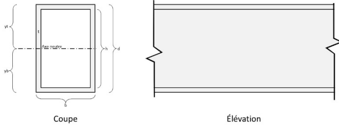
Situation #3 : Tube rectangulaire avec ZAT transversale à une face latérale
