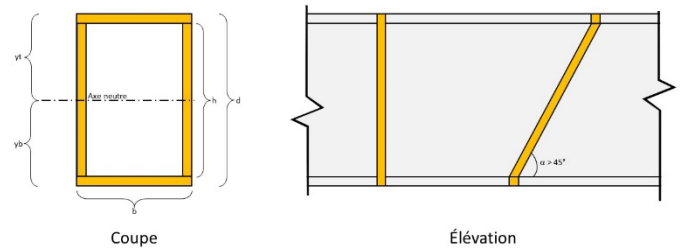
Situation #6 : Tubes rectangulaires assemblés avec soudures transversales (ou soudures obliques considérées comme transversales)
