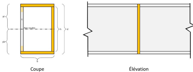
Situation #5 : Tube rectangulaire avec ZAT transversales à toutes les faces sauf à une face latérale
