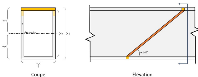
Situation #7 : Tubes rectangulaires assemblés avec soudures obliques Soudure transversale à une face horizontale
