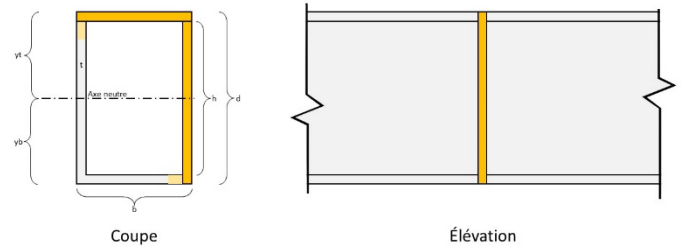
Situation #4 : Tube rectangulaire avec ZAT transversales à la face supérieure et une face latérale
