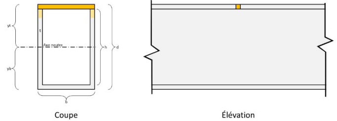
Situation #4 : Tube rectangulaire avec ZAT transversales à la face supérieure et une face latérale
